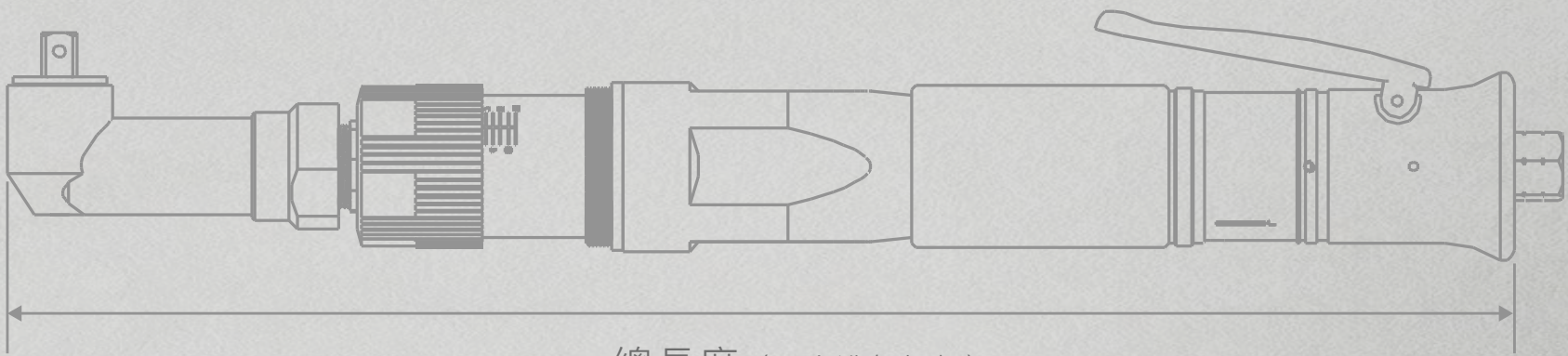
總長度（不含進氣螺帽）
